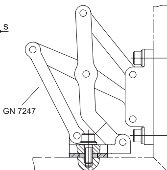
安装示例
